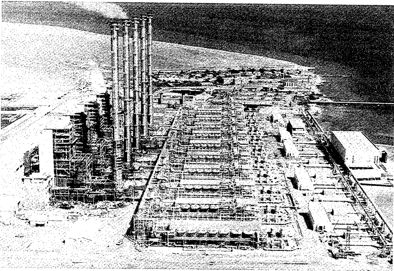
對 사우디아라비아 脫鹽水플랜트
